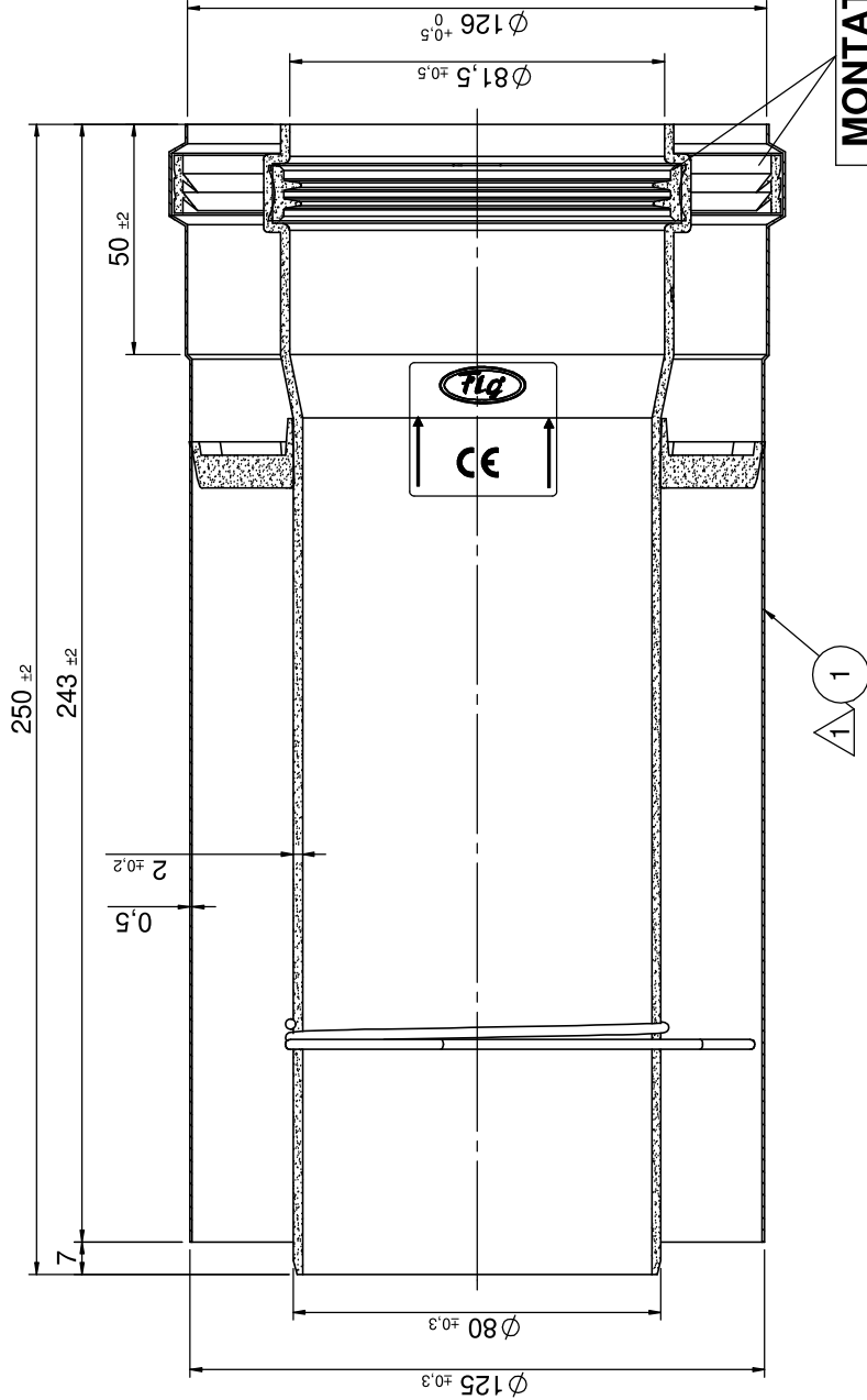
SEZ. A-A
